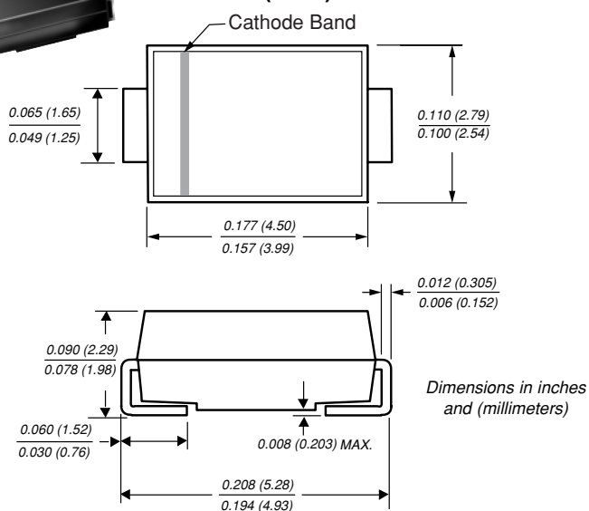
DO-214AC (SMA)
