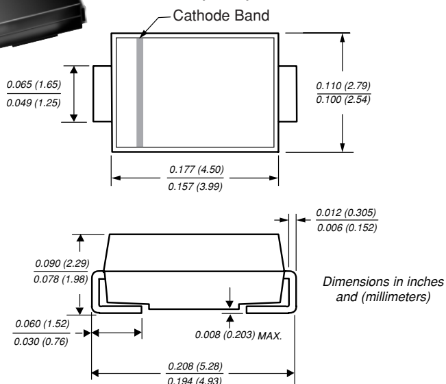
DO-214AC (SMA)
