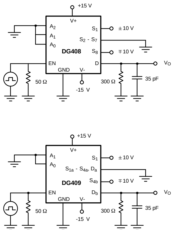
TEST CIRCUITS
