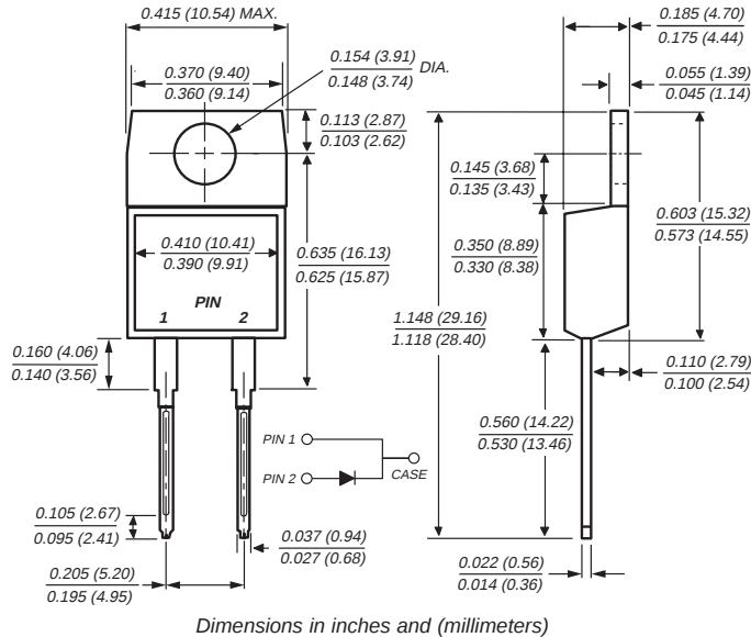
TO-220AC
