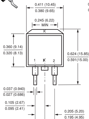
TO-263AB
