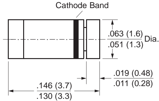
MiniMELF (SOD-80C)
