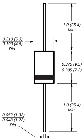
DO-201AD
