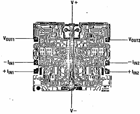
DIE SIZE: 85 x 71 MILS
