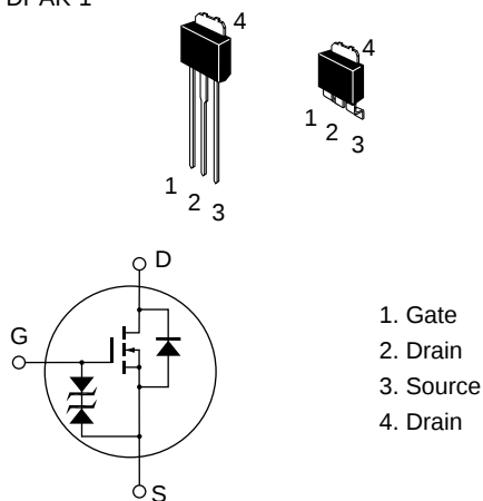
DPAK-1
