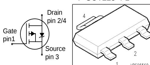
P-SOT223-4-1
