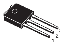
TO-251 IPAK (Suffix "-1")
