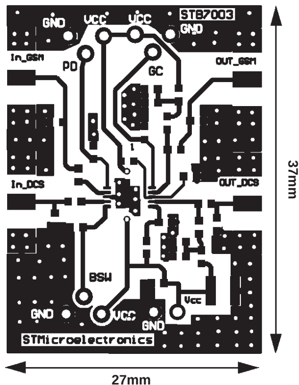
TOP LAYER
