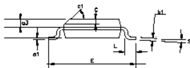
PowerSO-8
