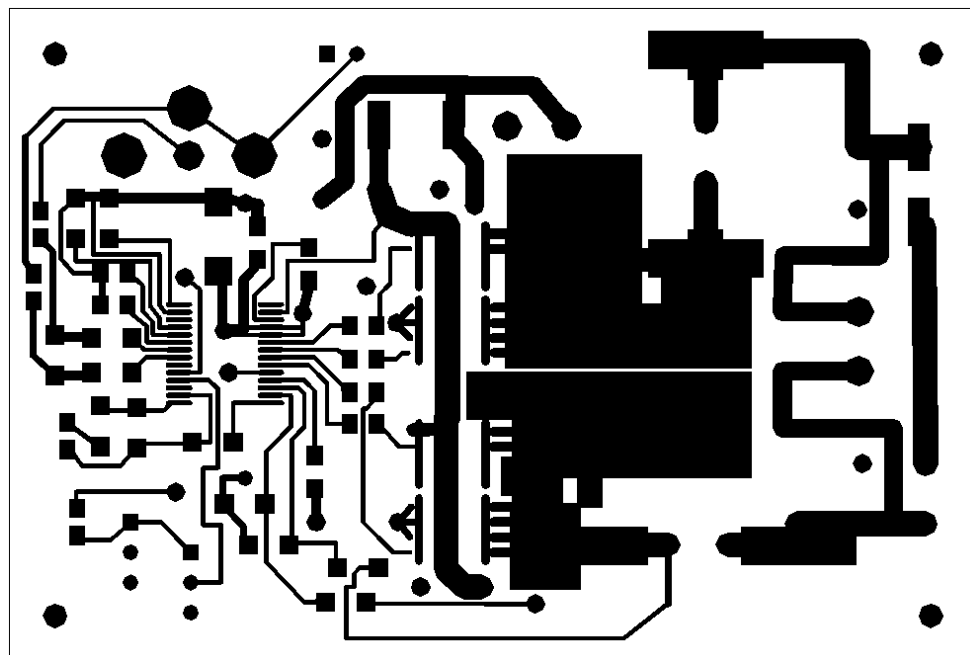
Top Layer
