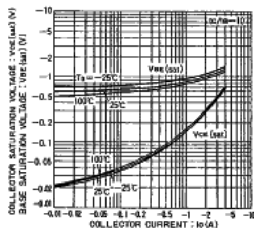
Fig.10 コレクタ・エミッタ間飽和電圧 —コレクタ電流特性
