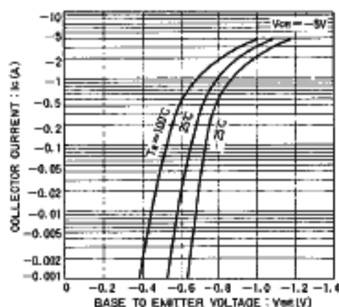
Fig.4 エミッタ接地伝達静特性
