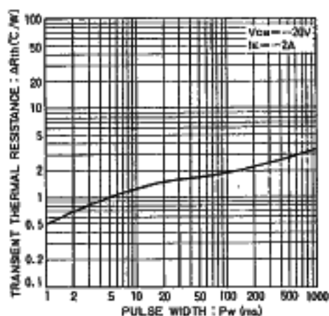
Fig.3 過渡熱抵抗
