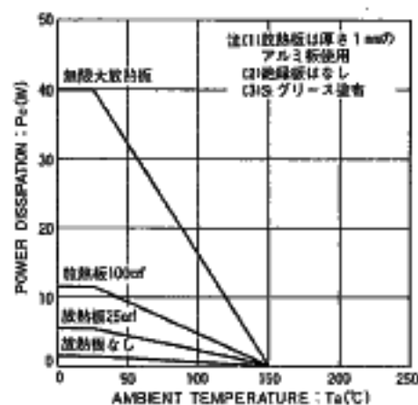
Fig.1 電力耗散曲線
