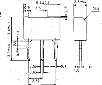
(1)エミッタ (2)コレクタ (3)ベース
