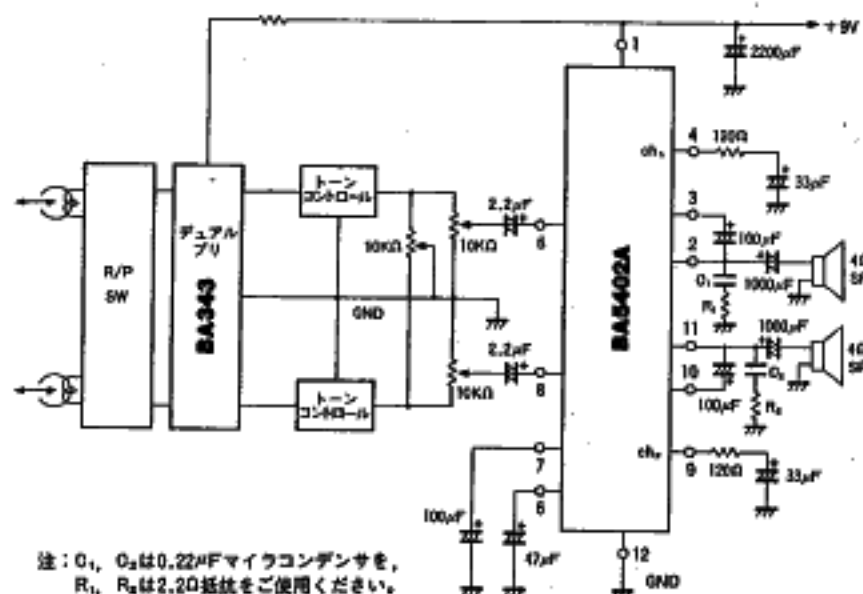
Fig. 2 テープレコーダへの応用回路例
