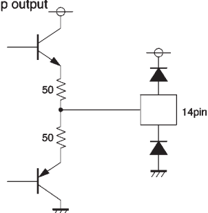
Op-amp output
