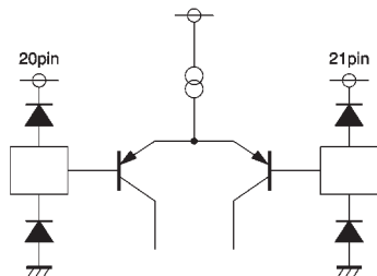
Op-amp input
