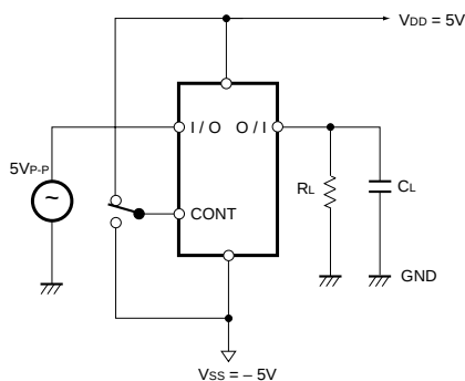
Fig. 2 (d) Sine wave distortion, feedthrough attenuation
