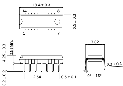
DIP14
