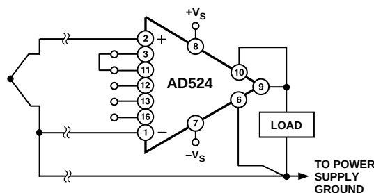
b. Thermocouple
