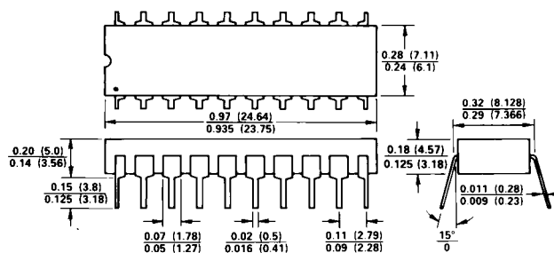
20-Pin Cerdip (Q-20)
