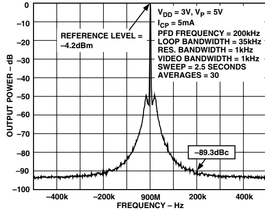
TPC 7. ADF4208 RF1 Reference Spurs (900 MHz, 200 kHz, 35 kHz)
