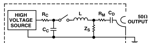
Figure 12. EFT Generator
