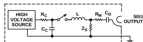
Figure 21. EFT Generator
