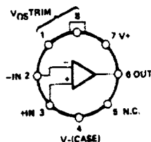
TO-99 (J-Suffix)
