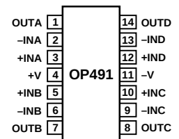
14-Lead SO (S Suffix)
