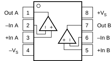
SO-8, PSO-8
