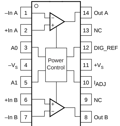
PSO-14
