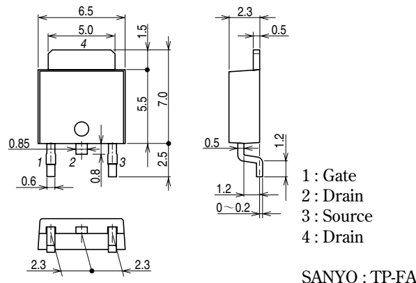
外形図 2092B (unit : mm)
