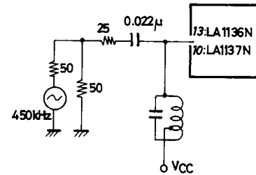
Detector input
