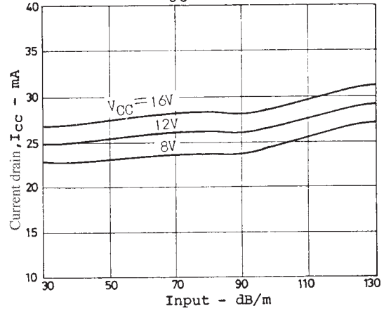
I_{CC} - Input
