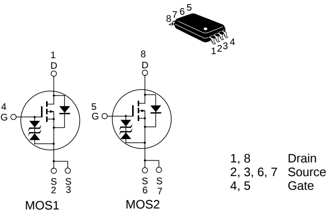
TSSOP-8
