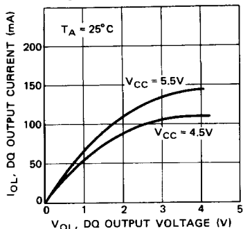
Fig. 30 – DQ OUTPUT CURRENT vs DQ OUTPUT VOLTAGE
