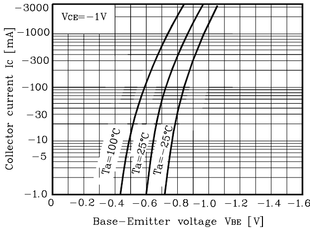
Fig. 2 I_C - V_{BE}
