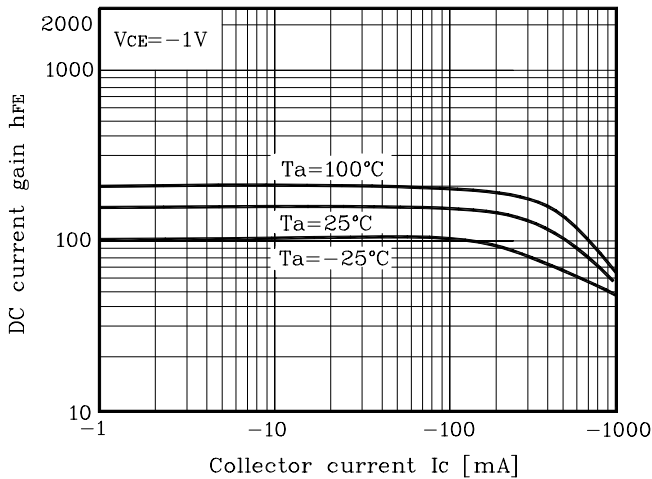
Fig. 4 h_{FE} - I_C
