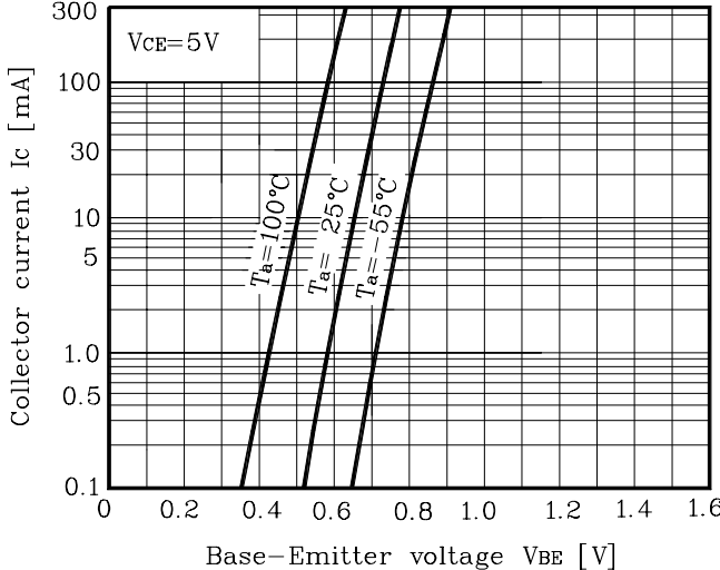
Fig. 2 I_C - V_{BE}
