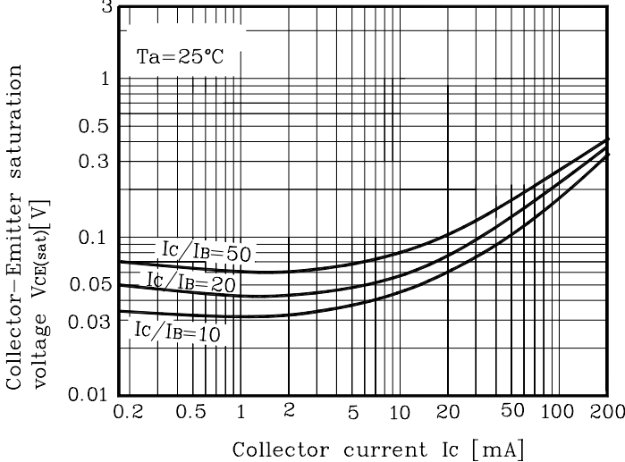
Fig. 5 V_{CE(sat)} - I_C
