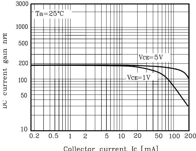
Fig. 4 h_{FE} - I_C
