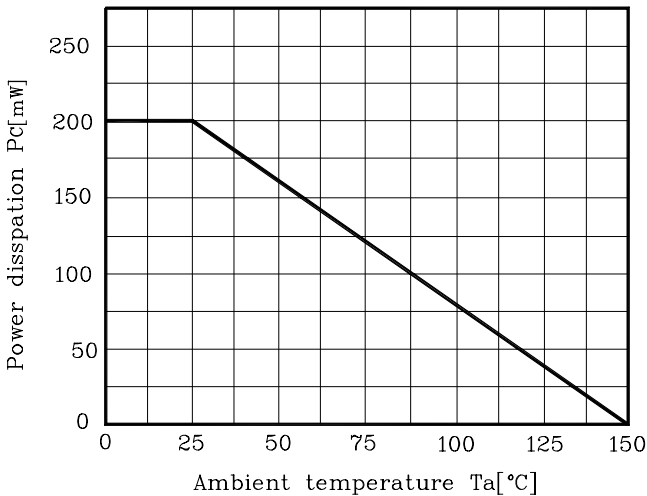
Fig. 1 P_C - T_a
