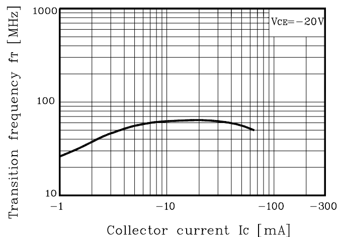
Fig. 3 f_T - I_C
