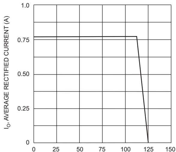
T_L , LEAD TEMPERATURE (°C)
