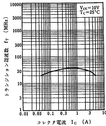
f_T - I_C
