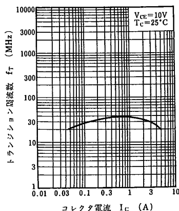
f_T - I_C
