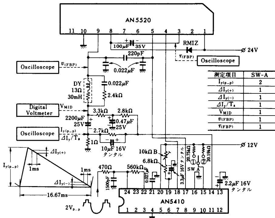
Test Circuit 1 ( I_{y(p-p)} , \Delta I_{y(+)} , \Delta I_{y(-)} , \Delta I_y / T_a , V_{MID} , v_{(FBP)} , \tau_{(BLP)} )
