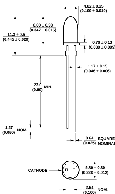
HLMP-8102/-8103
