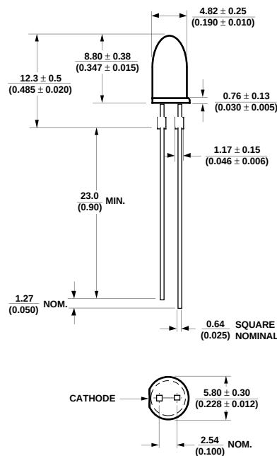
HLMP-8100
