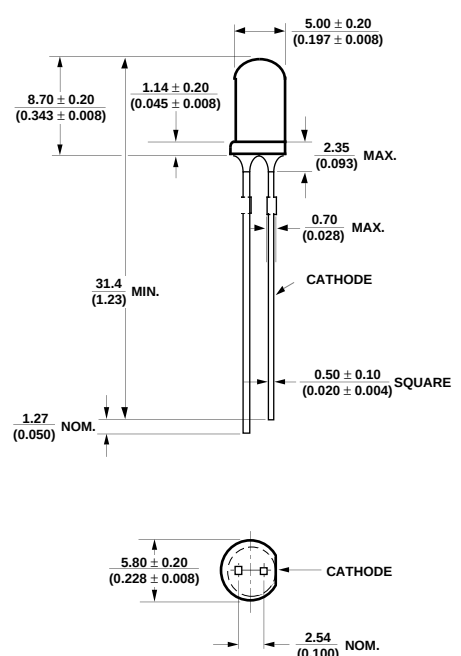
HLMP-C100/-C110
