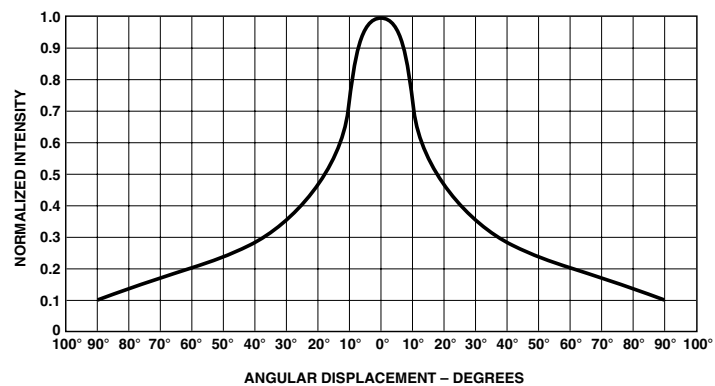
Figure 9. HLMP-Q102/-Q152
