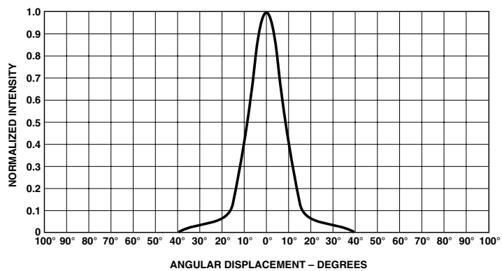
Figure 8. HLMP-Q106/-Q156.
