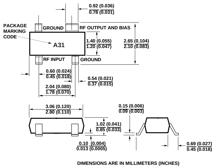
SOT-143
