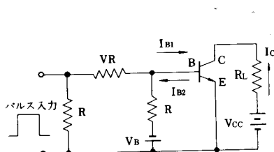
スイッチング特性測定回路
