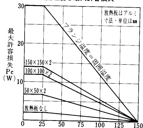
周囲温度と最大許容損失
