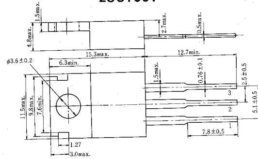
2SC1061
