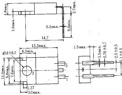
2SC1060
