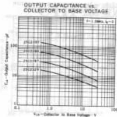
2SC2329
