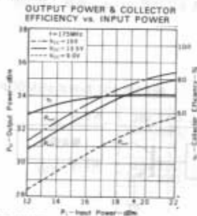
2SC2287
