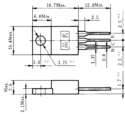
外形寸法 (単位: mm)
