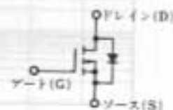
電極接続
