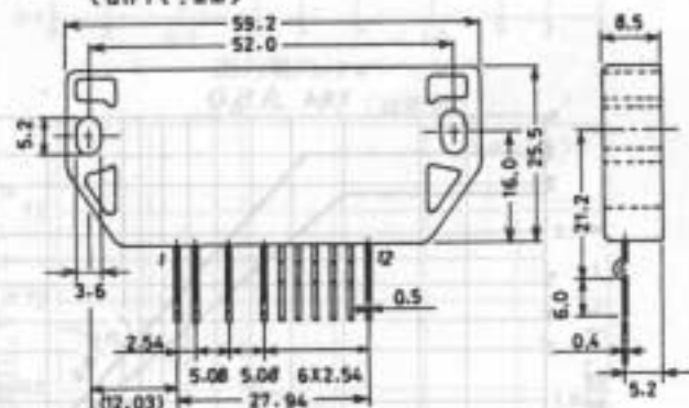
外形圖 4055 (單位:mm)
